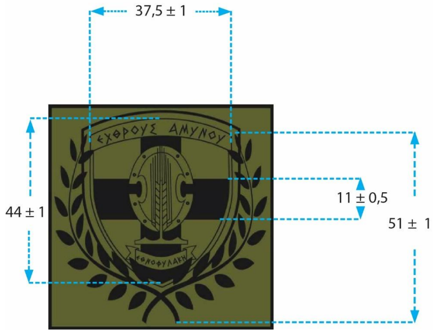
Εικόνα 5. Διαστάσεις Σχεδίου Διακριτικού 15 ετών
