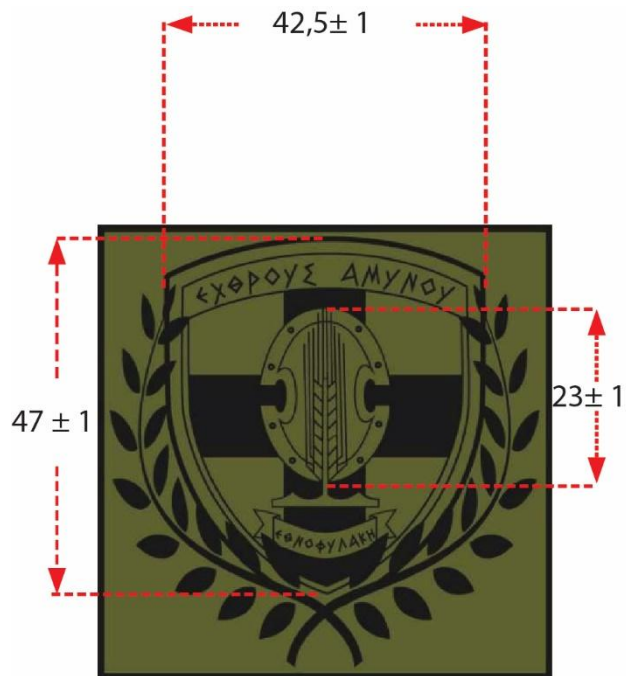
Εικόνα 6. Διαστάσεις Σχεδίου Διακριτικού 15 ετών
